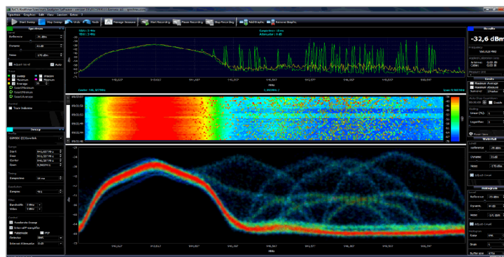
Visualisation d'un signal GSM perturbé
