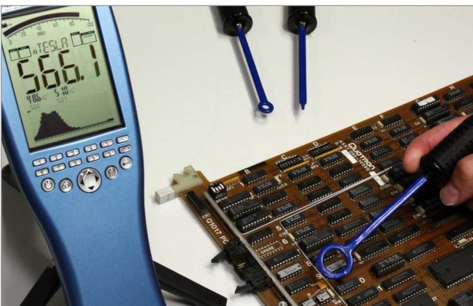
Mesure sur un composants électroniques avec le SPECTRAN NF-5030 et le set de sondes de champ proche Aaronia PBS 2
