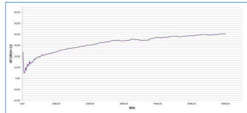
Facteur d'antenne HyperLOG 20600 EMI
