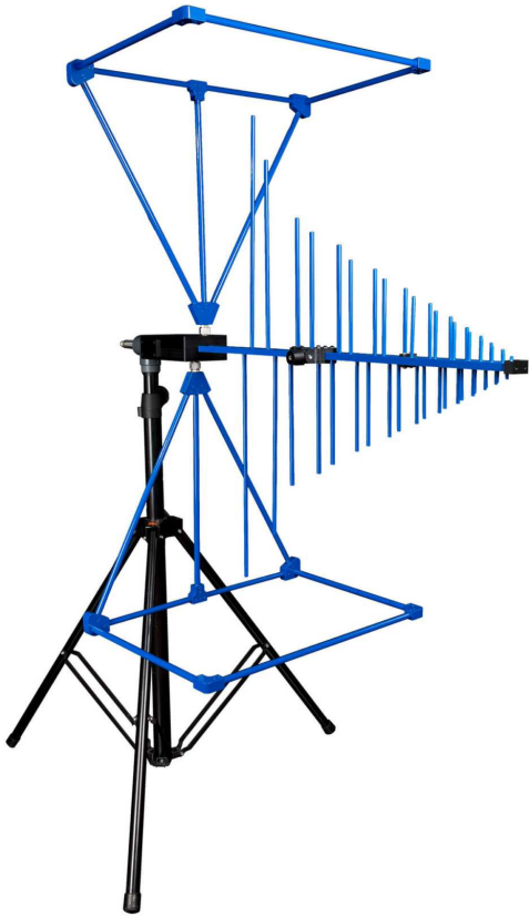
Antenne HyperLOG EMI avec trépied optionnel
