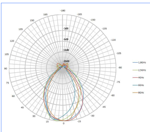
Pattern horizontal Série HyperLOG 30 X
