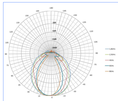
Pattern vertical Série HyperLOG 30 X
