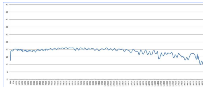
Diagramme de gain HyperLOG 30200X
