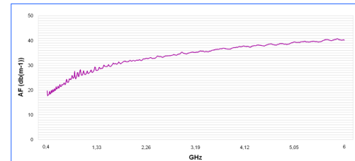
Facteur d'antenne HyperLOG 4060
